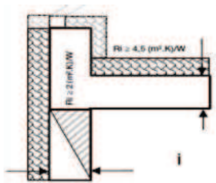
Isolation des acrotères
