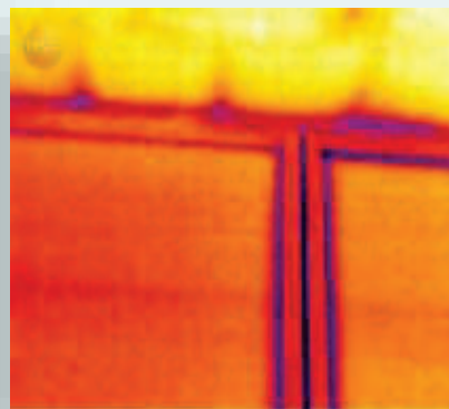
Mur intérieur non isolé Déperditions de chaleur et fuites d'air Violet = froid de l'extérieur qui rentre à l'intérieur
