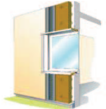
Isolation des façades en partie courante avec un système d'isolant sous enduit mince
