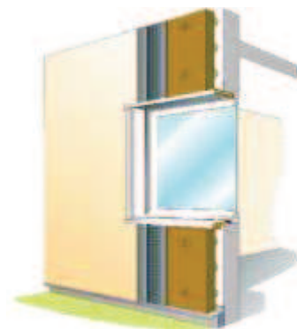
Isolation des façades en partie courante avec un système d'isolant sous enduit mince
