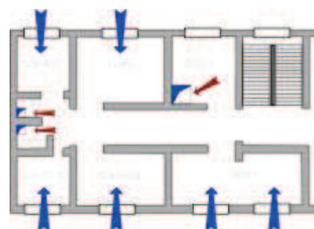
Entrée d'air hygroréglable
