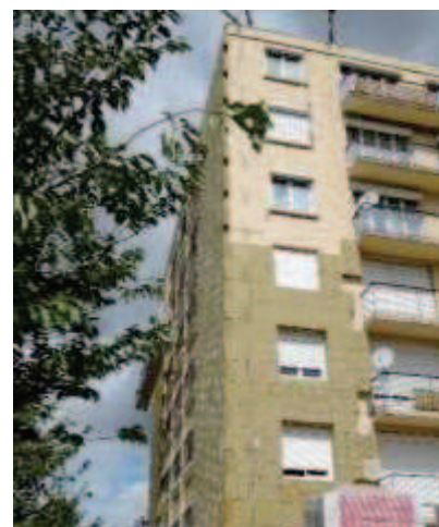
Isolation avec de la laine de roche
