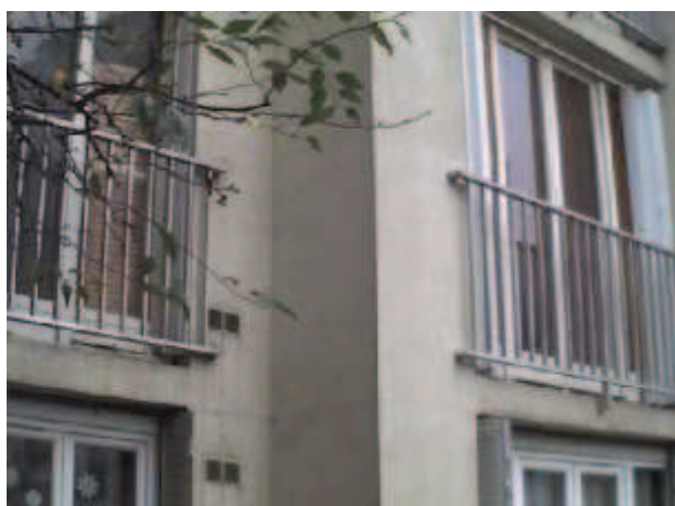
Mise en évidence d'un pont thermique au niveau du mur de refend
