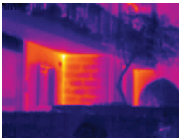
Mise en évidence des rangées de parpaings non isolées
